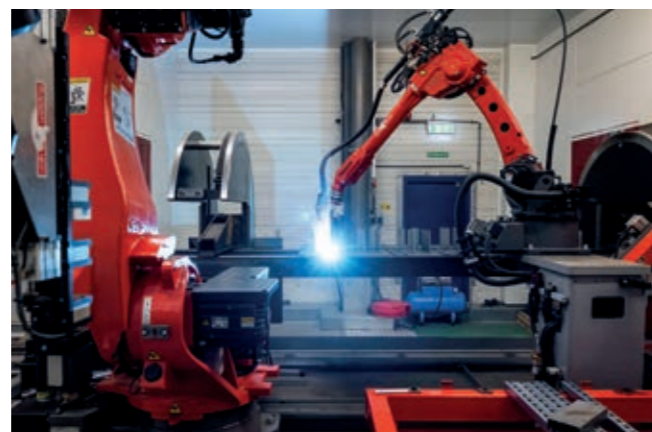
ROBOTLASSEN
