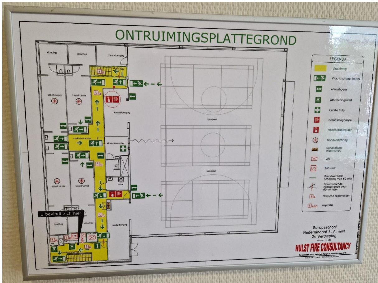
2 e etage ( gymzaal) Nederlandhof 3
