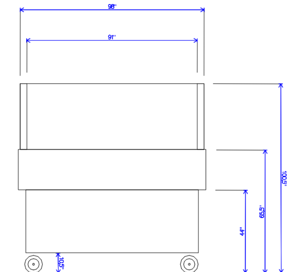
Vooraanzicht RVS Koeltafel 1000
