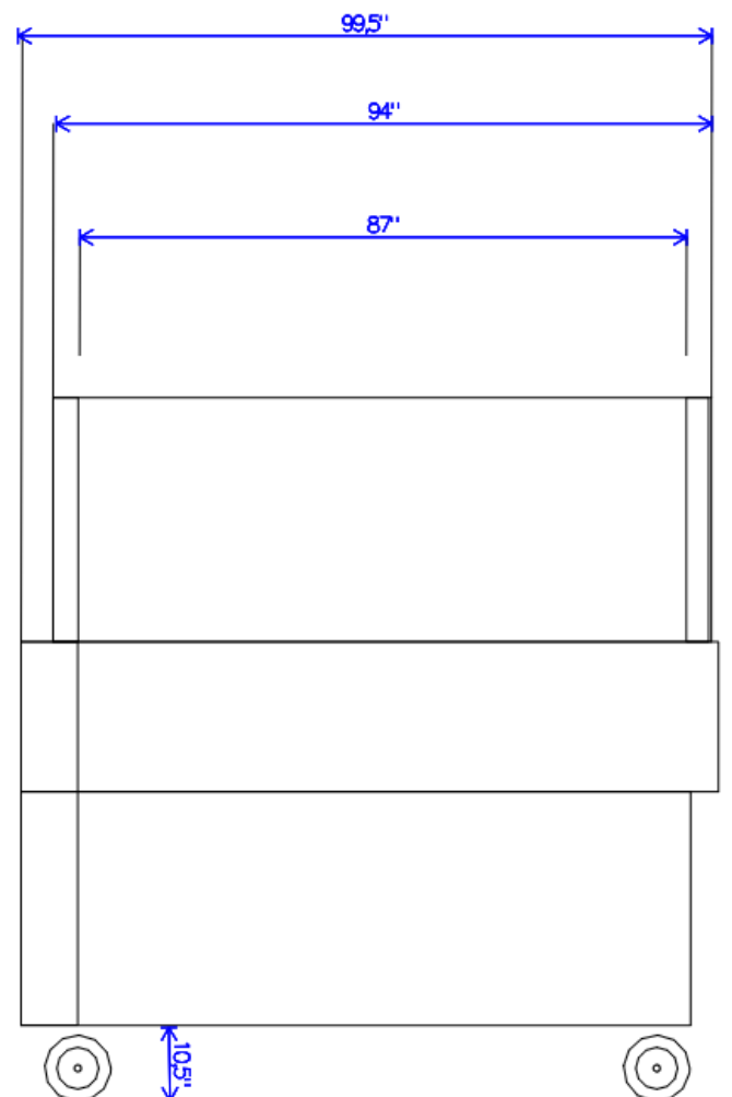
Zijaanzicht RVS Koeltafel
